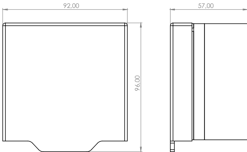
Műszaki rajz az opcionálisan megvásárolható védőfedéllel
