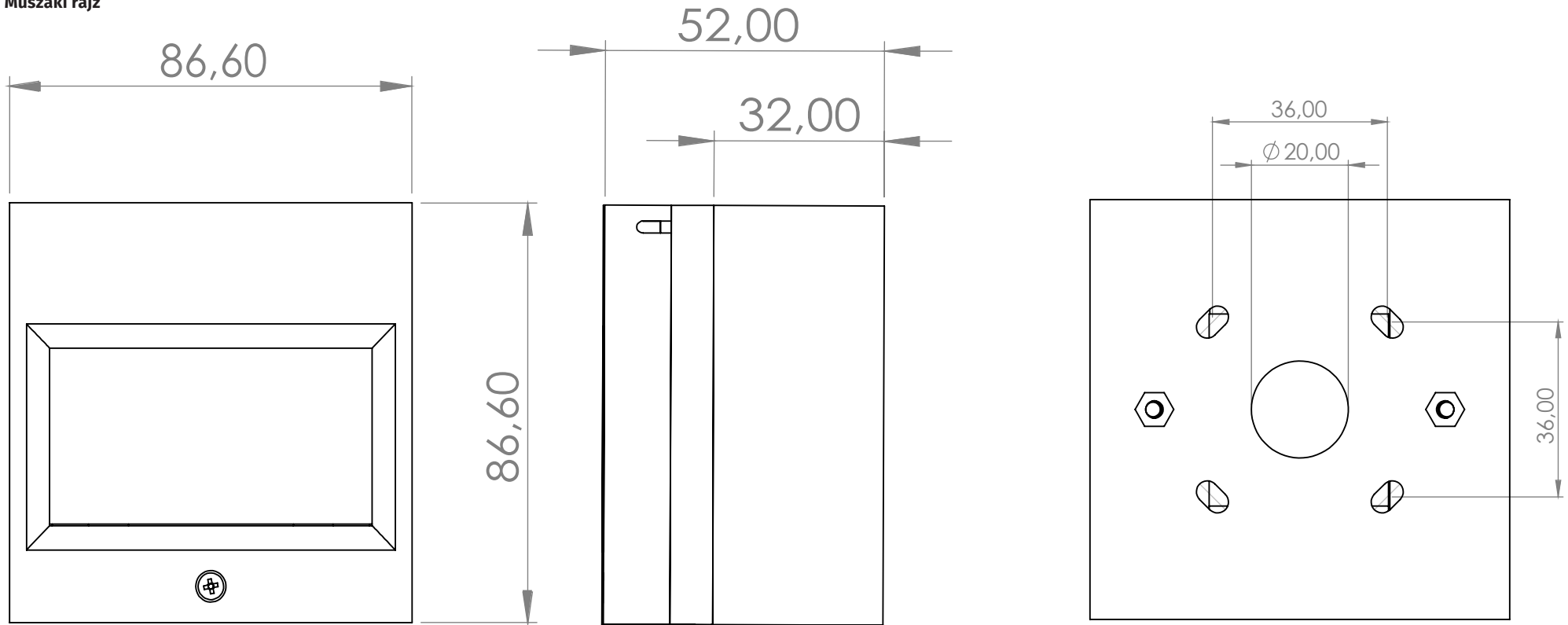
Műszaki rajz
